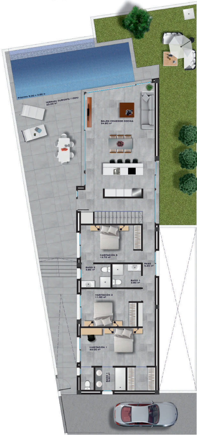
PLANTA BAJA. 1/100
